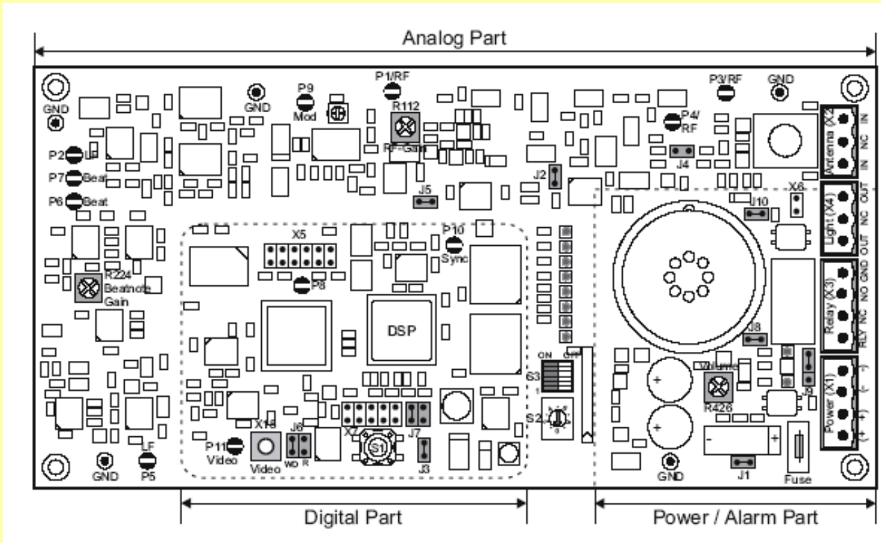
Фиг.3. Плата приемника
