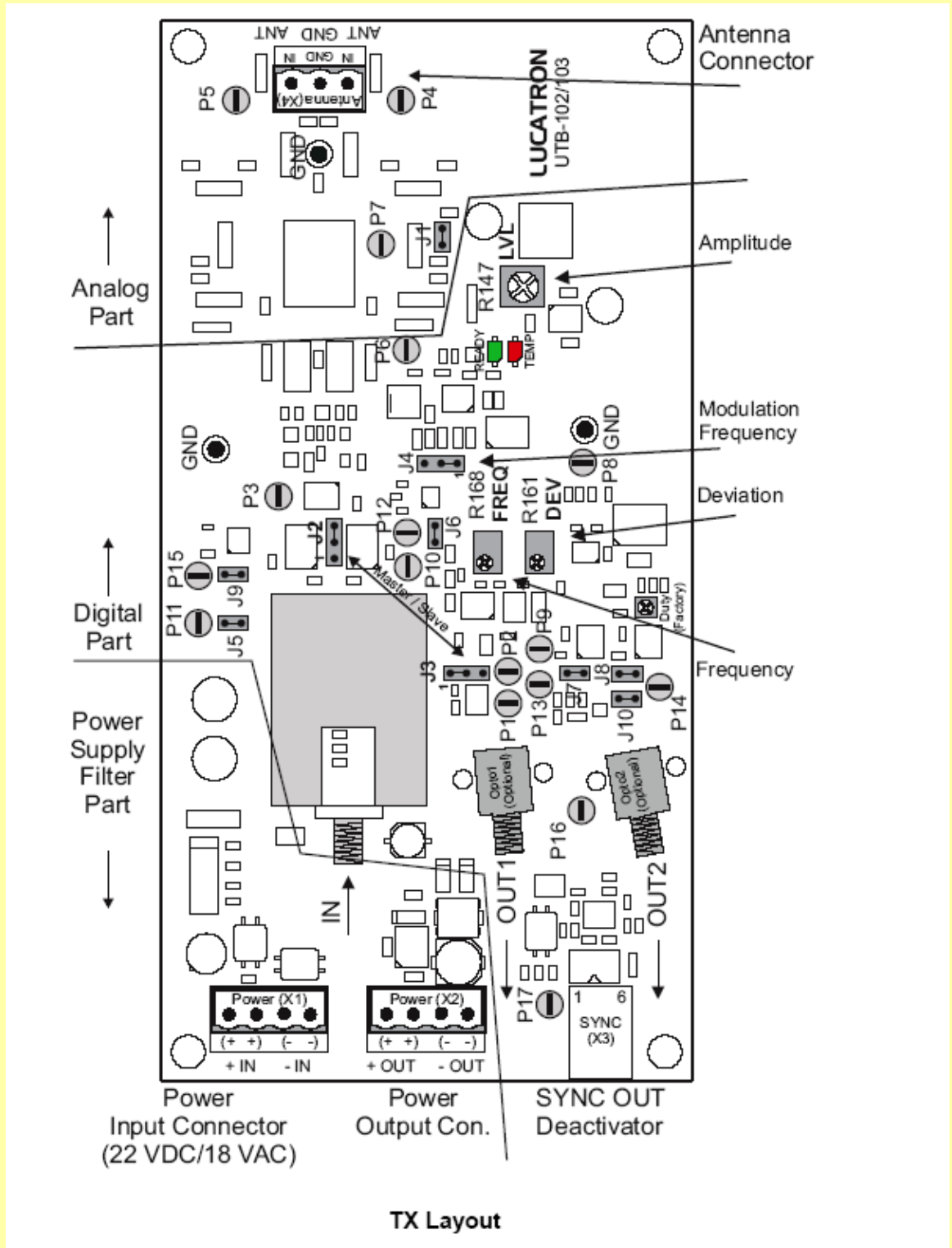
Фиг.1. Плата передатчика UTB-102/103
